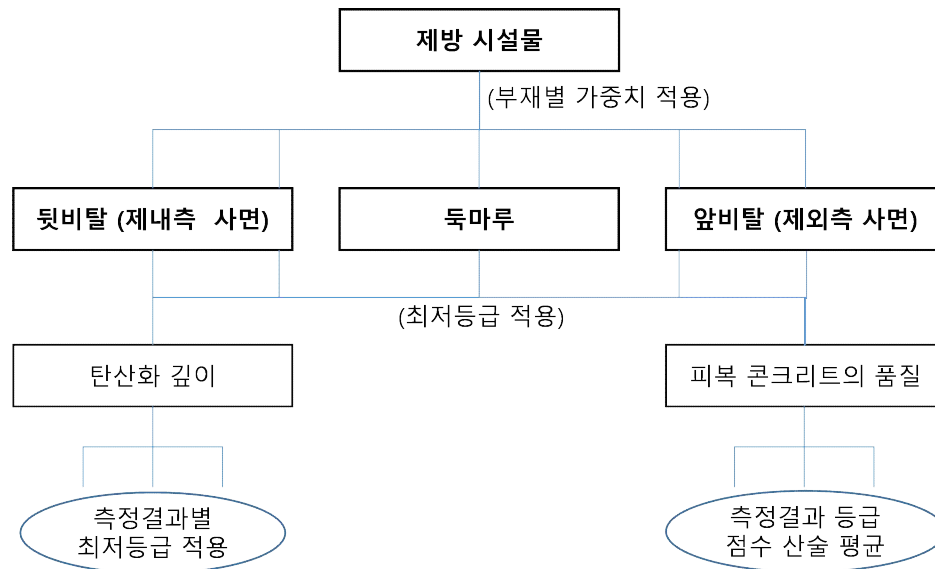
[그림 8.2] 제방의 내구성능 평가 예시
